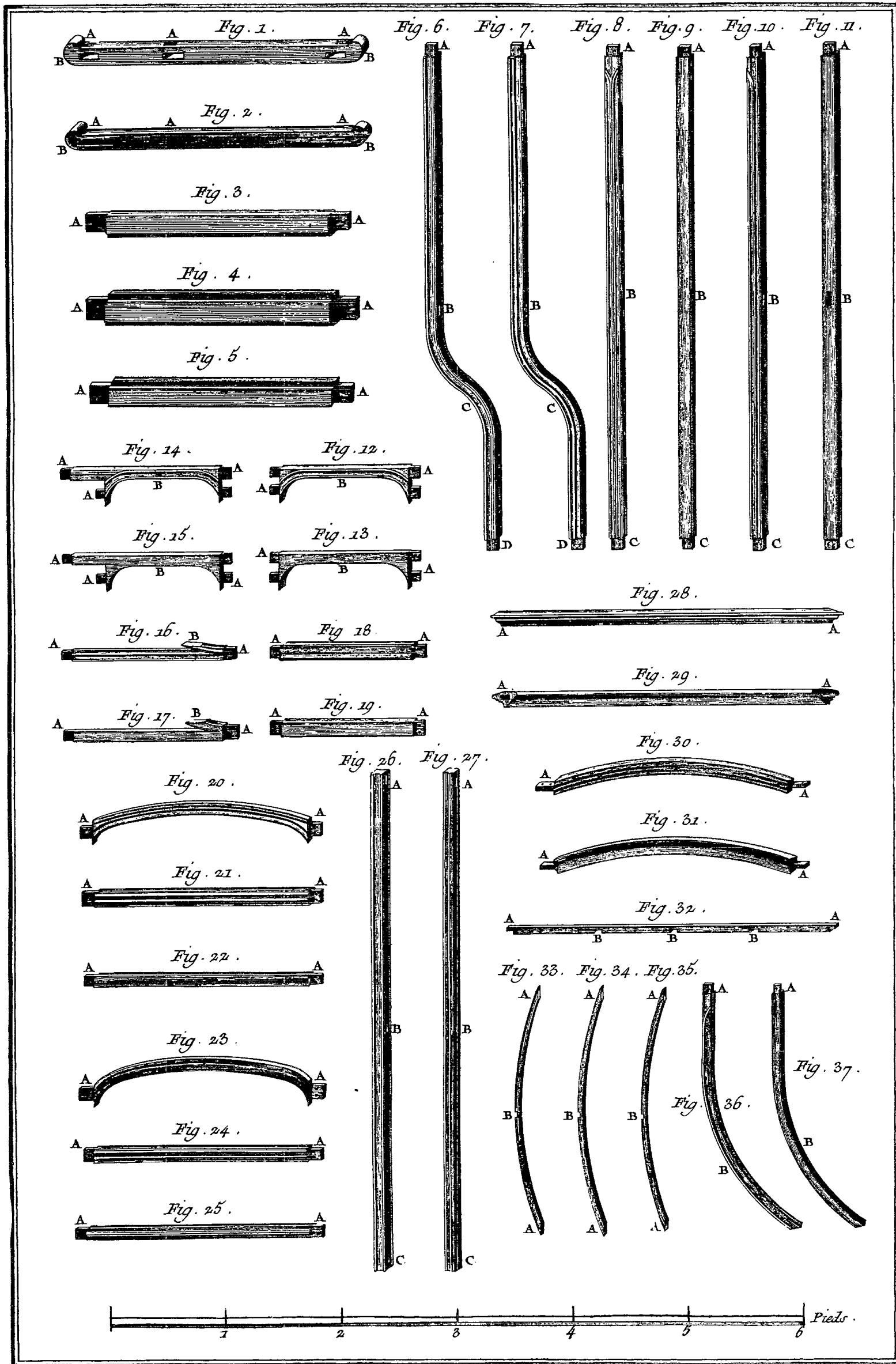
Menuisier en Voitures, Chaise à Porteur, Détails.
