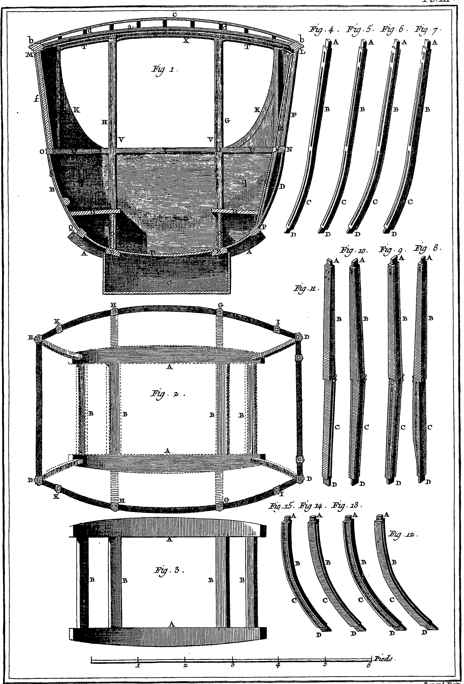
Menuisier en Voitures, Berline a la Francaise, Détails.
