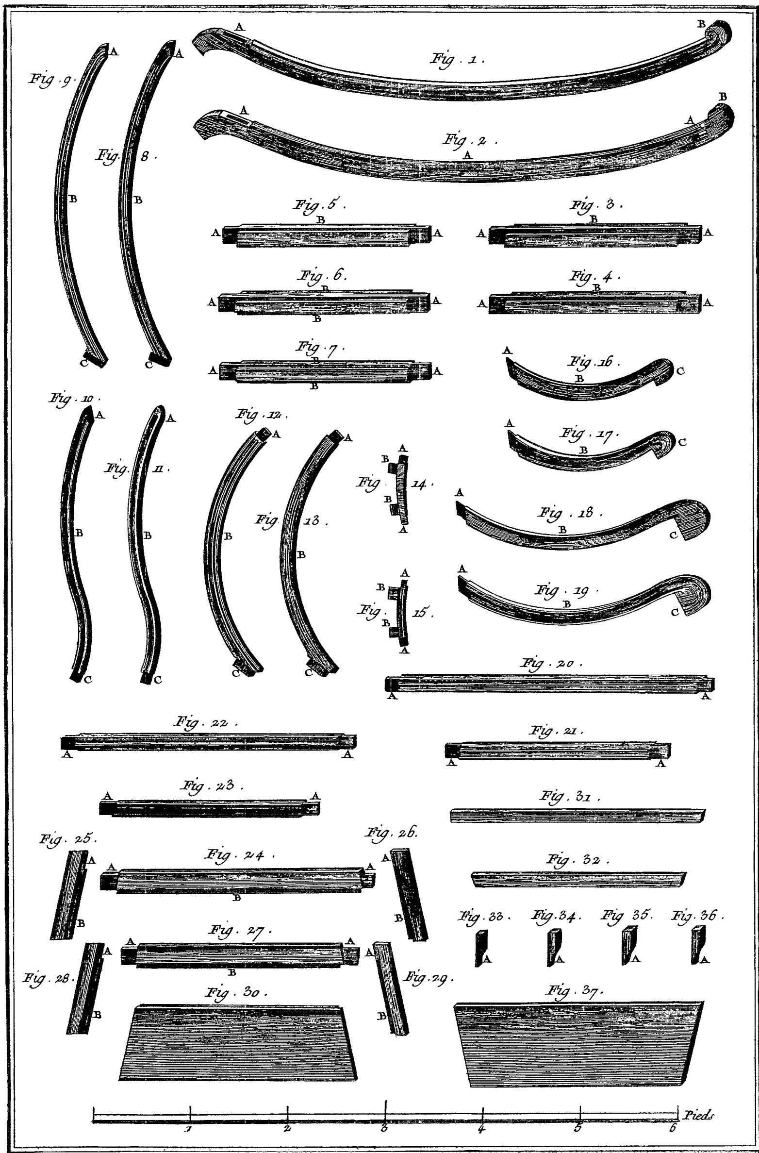
Menuisier en Voitures, Carosse de Jardin à 4 places, Détails.
