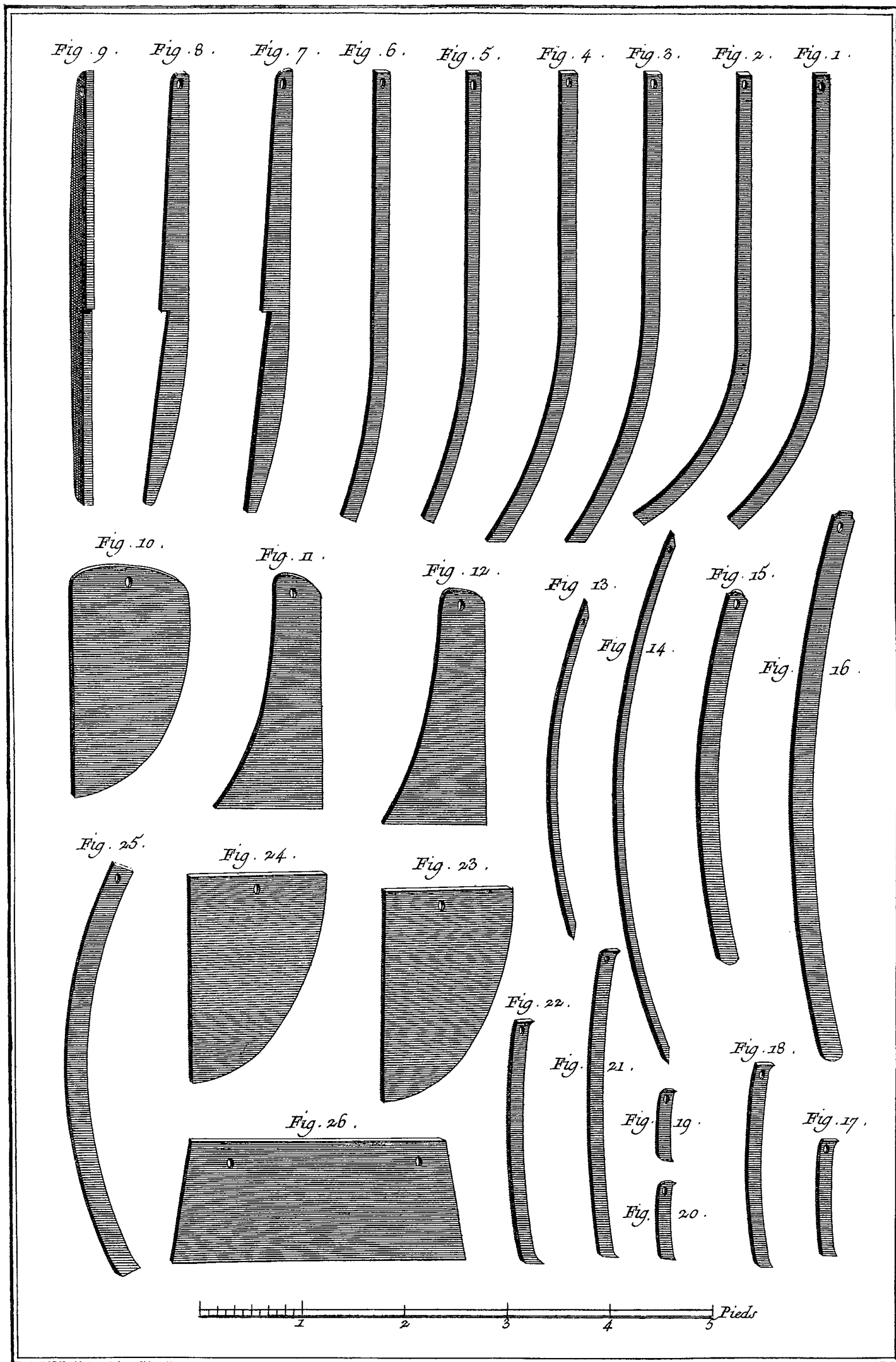
Menuisier en Voitures, Outils Calibres.
