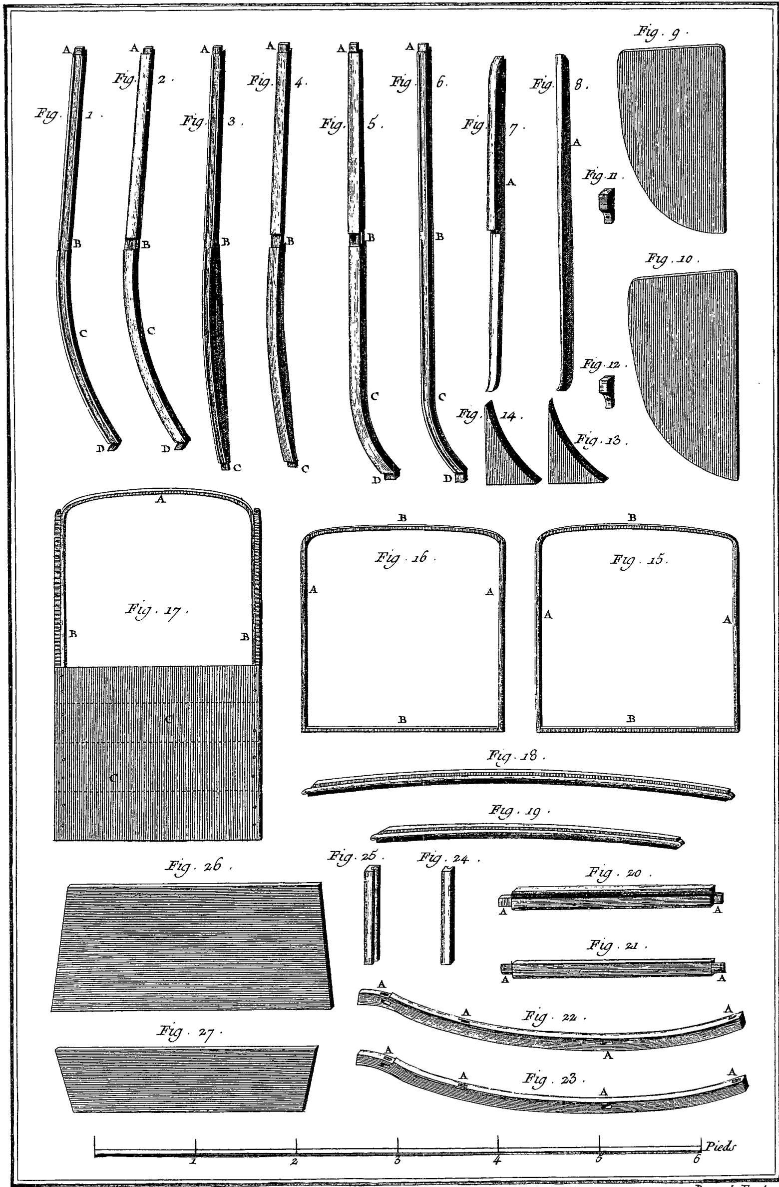
Menuisier en Voitures, Diligence à l'Anglaise, Détails.
