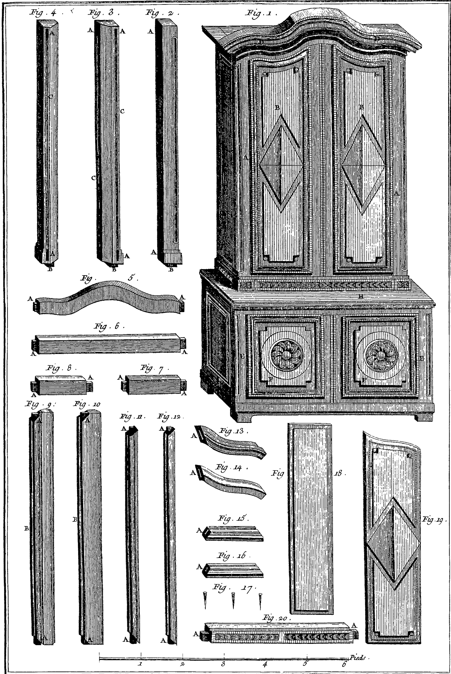
Menuisier en Meubles, Buffet.
