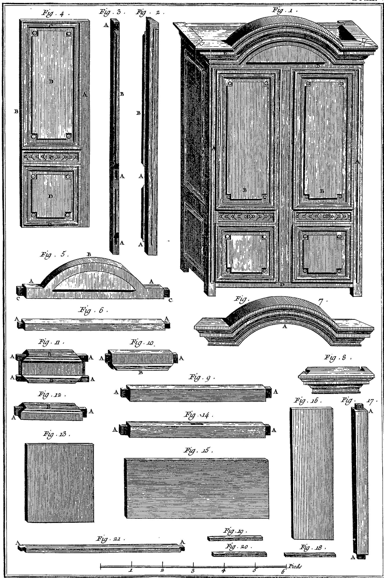
Menuisier en Meubles, Armoire.
