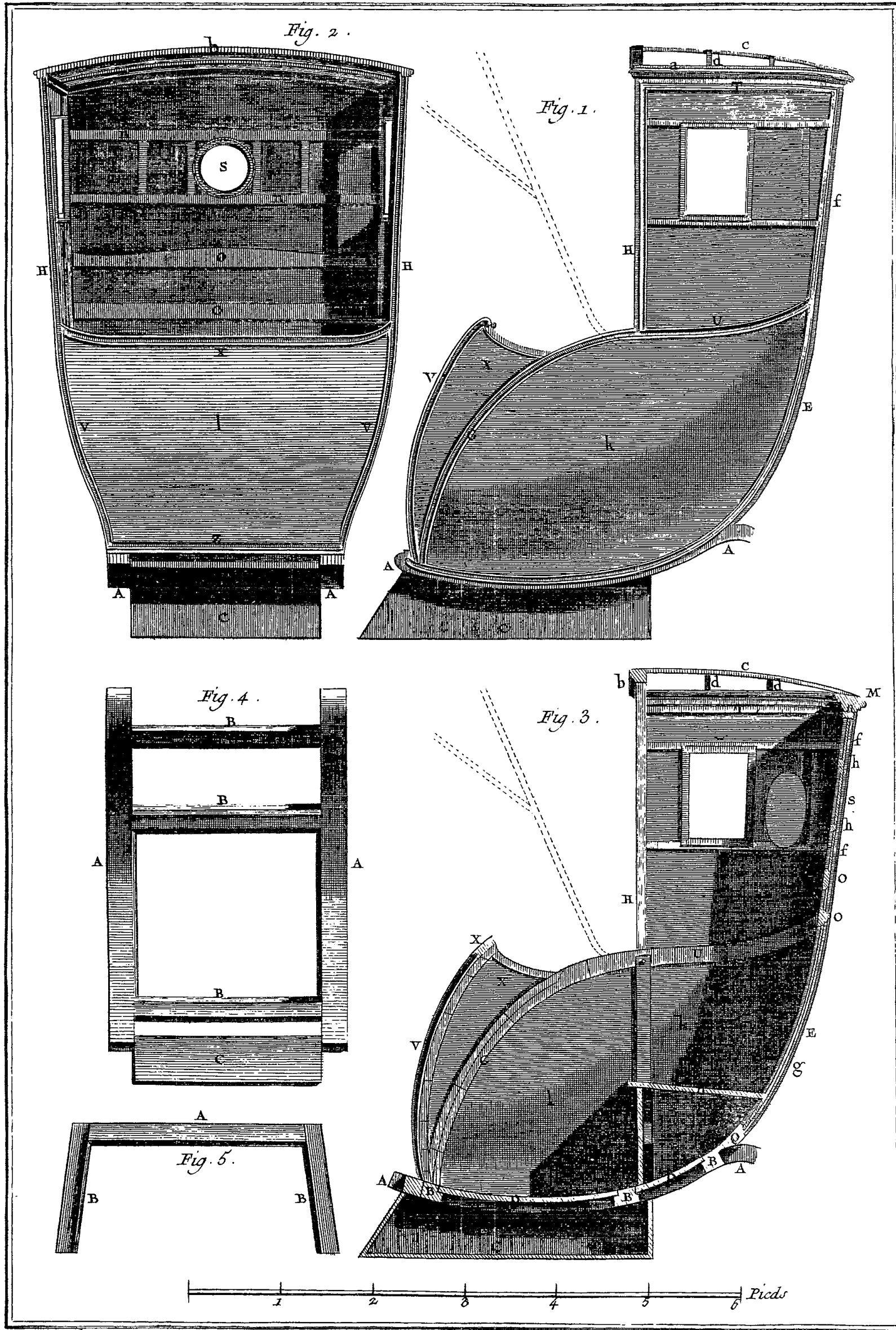
Menuisier en Voitures, cabriolet.
