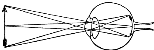
Fig. 3. — Trajet de la lumière dans l'œil.
