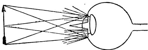
Fig. 2. — Trajet de la lumière dans l'œil.
