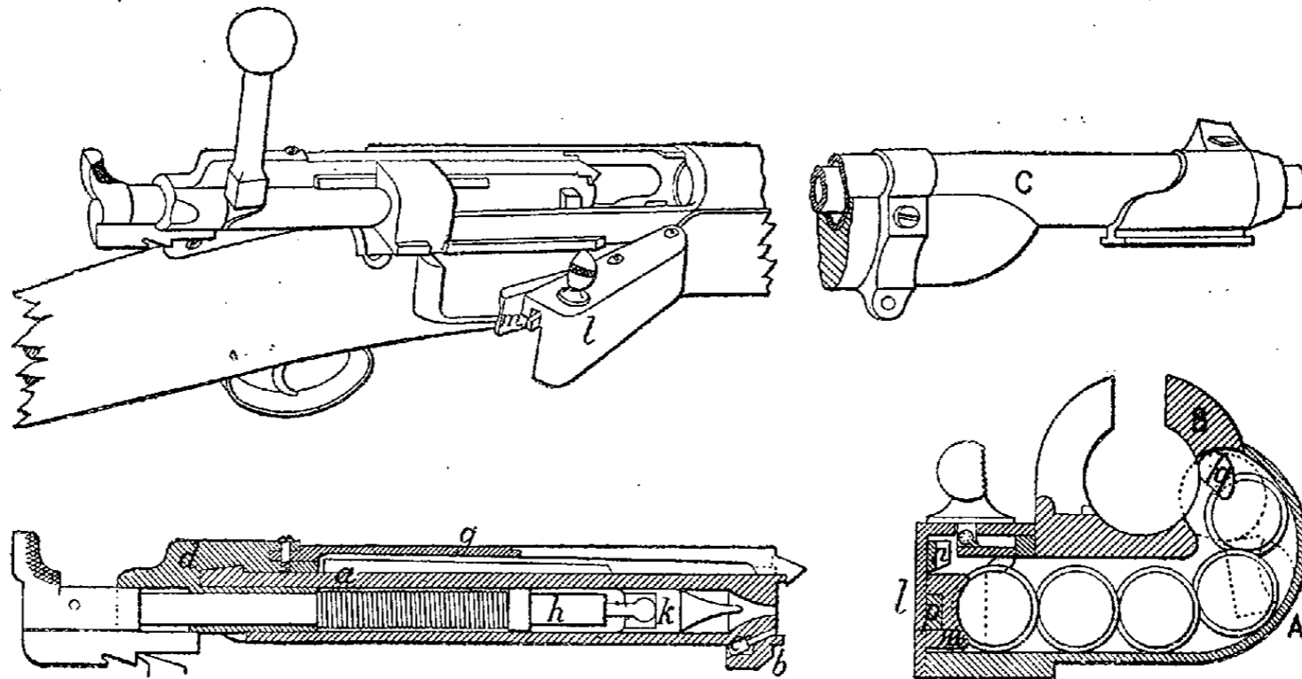
Fig. 17. — Fusil danois Krag-Jørgensen, modèle 1889.
