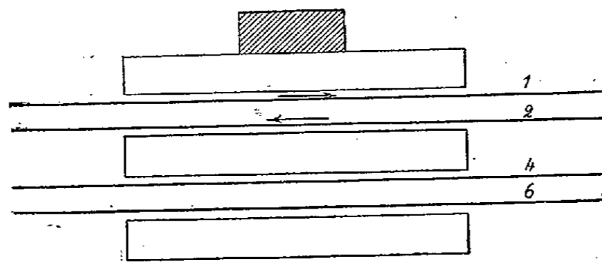
Fig. 3. — Transit-voyageurs pour quatre branches.
