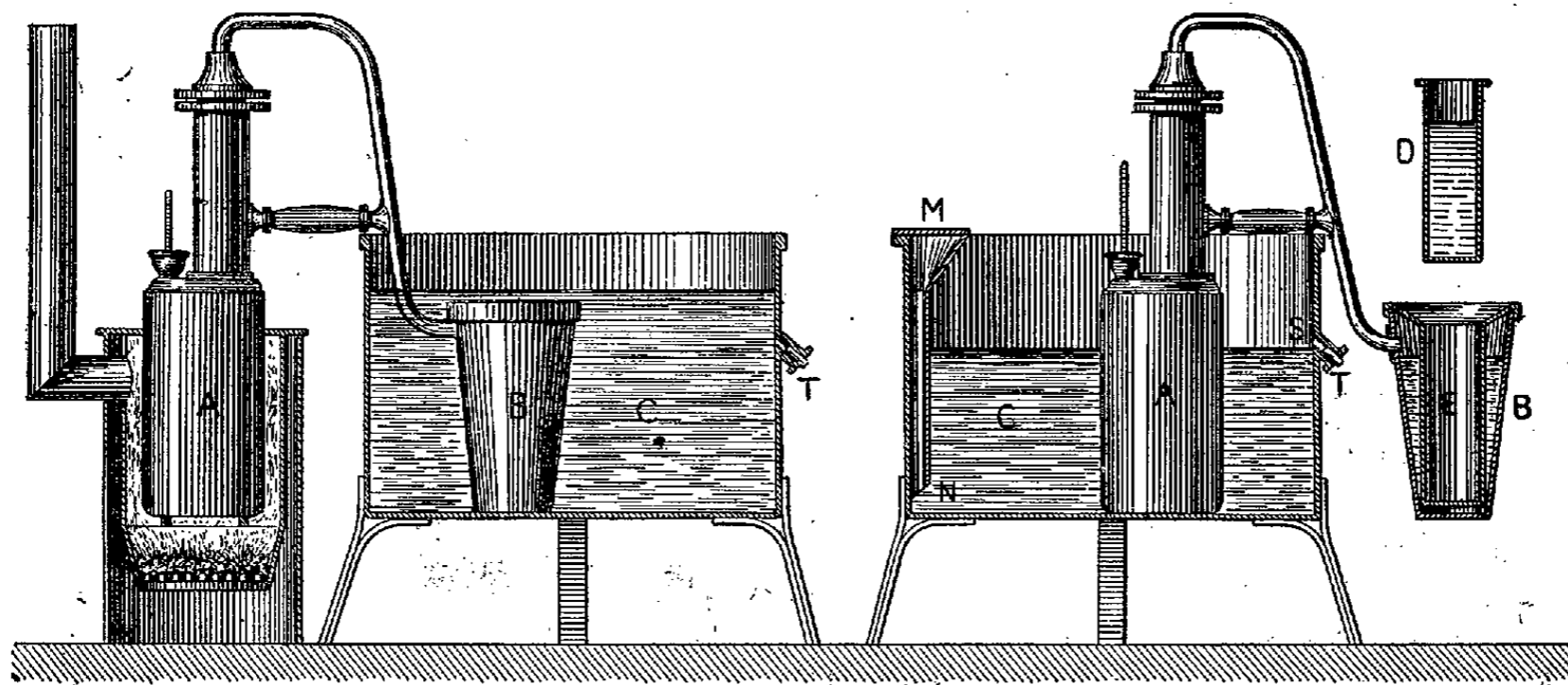
Fig. 4 et 5. — Appareil Carré.
