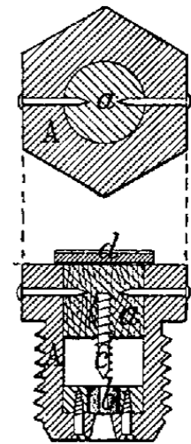
Fig. 1. — Fusée Desmarests.
