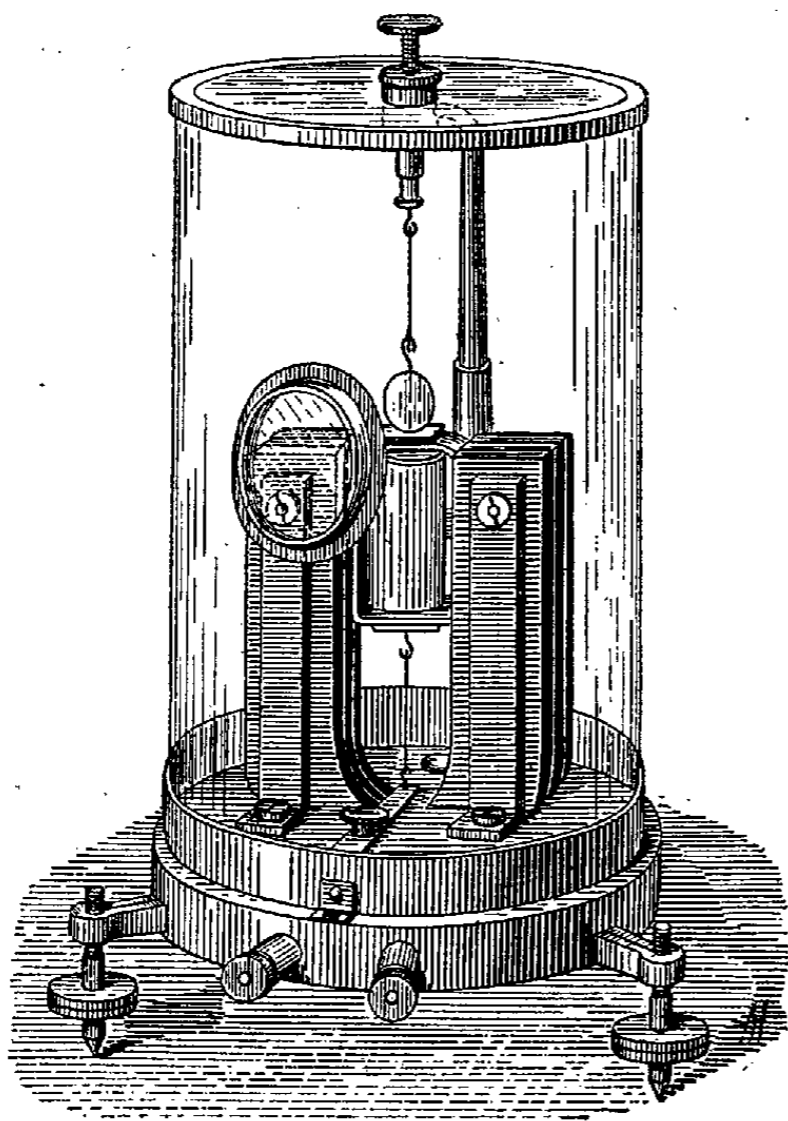
Fig. 3. — Galvanomètre de Desprez et d'Arsonval.]
