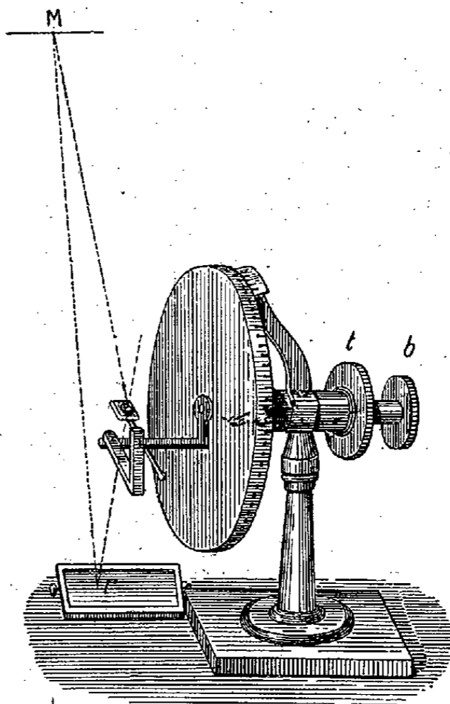
Goniomètre de Wollaston.
