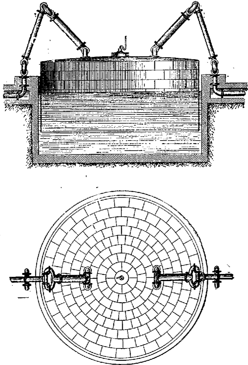
Gazomètre de Pauwels (coupe et plan).
