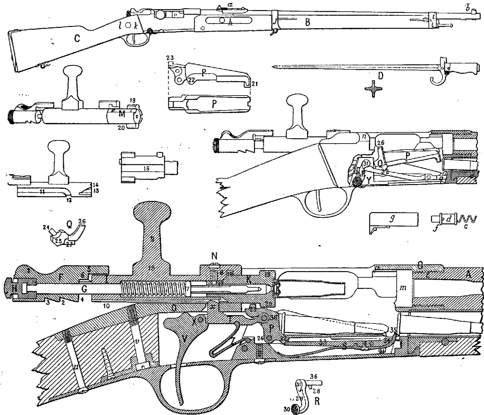
Fig. 12. — Fusil français, modèle 1886.
