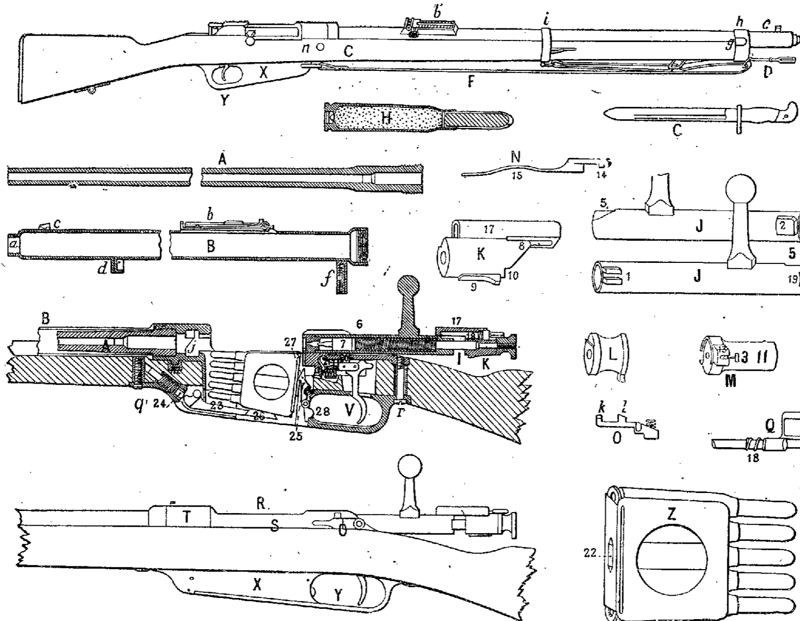
Fig. 13. — Fusil allemand, modèle 1888.
