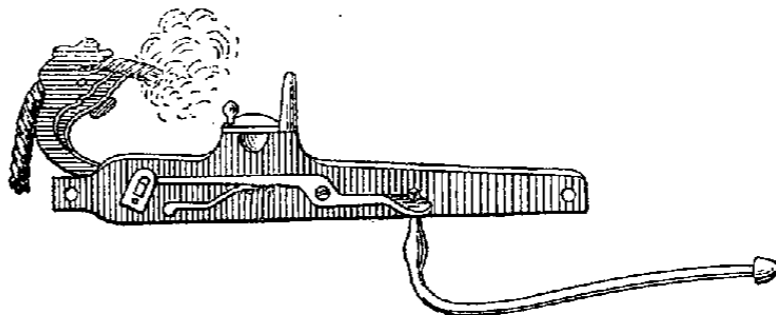
Fig. 4. — Platine à mèche.
