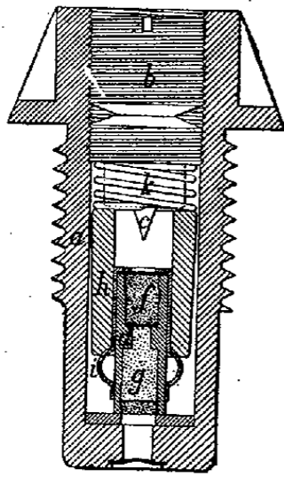
Fig. 2. — Fusée percuteur Budin. — a, corps de fusée qui se visse dans l'œil du projectile; b, bouchon; c, rugueux; d, percuteur porte-amorce; f, fulminate; g, poudre; h, masselotte; i, ressort d'armement; k, ressort de sûreté.
