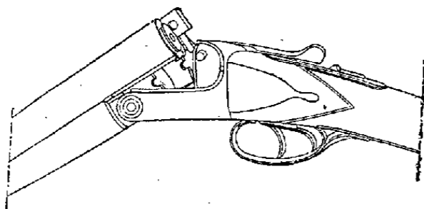
Fig. 21. — Fusil dit Hammerless.
