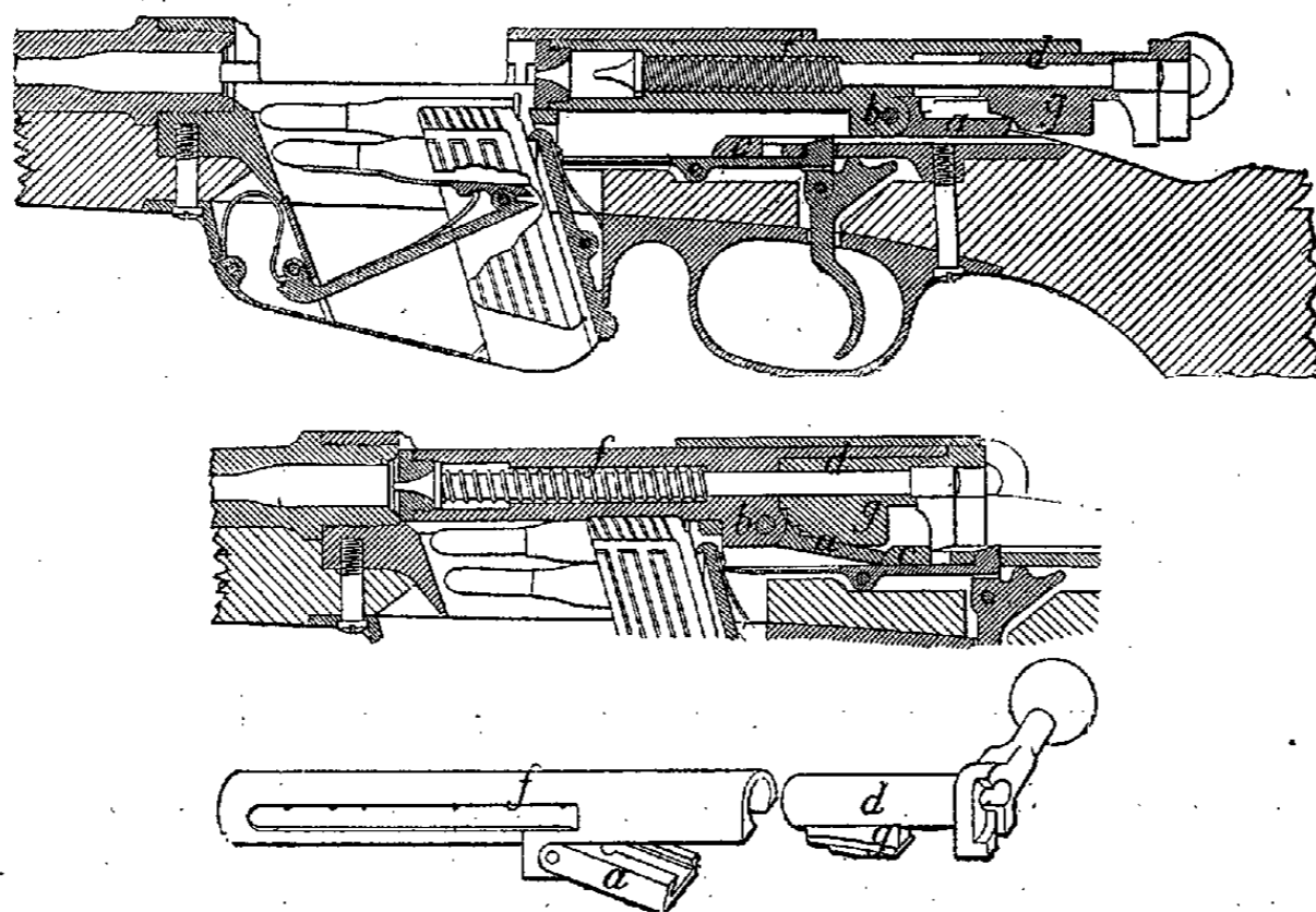
Fig. 15. — Fusil autrichien Mannlicher, modèle 1888-90.
