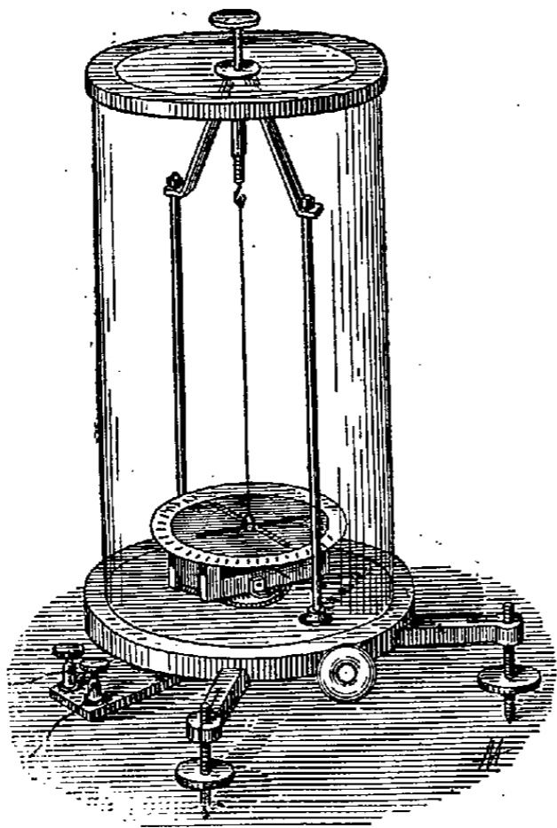
Fig. 1. — Galvanomètre de Nobili.
