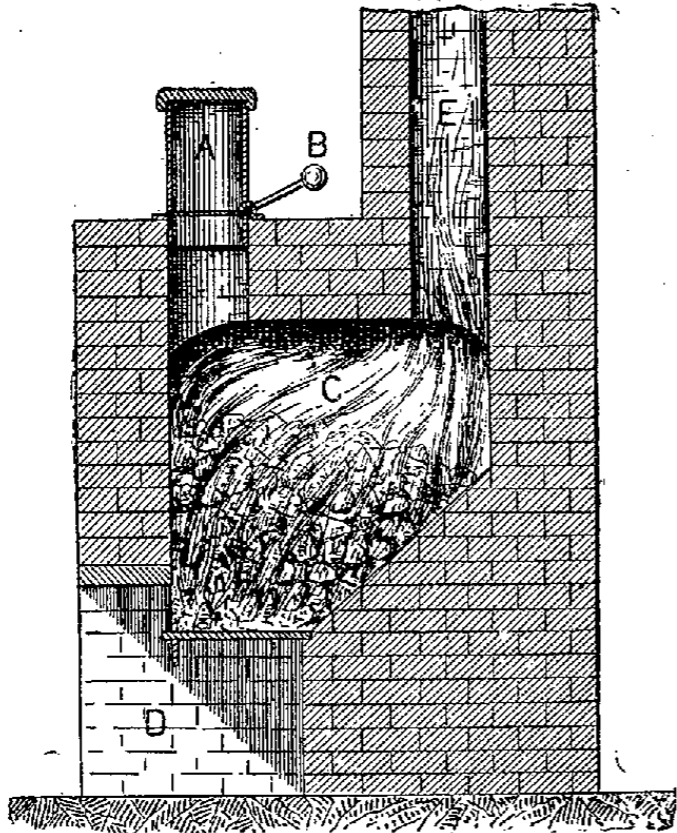
Coupe théorique d'un gazogène.
