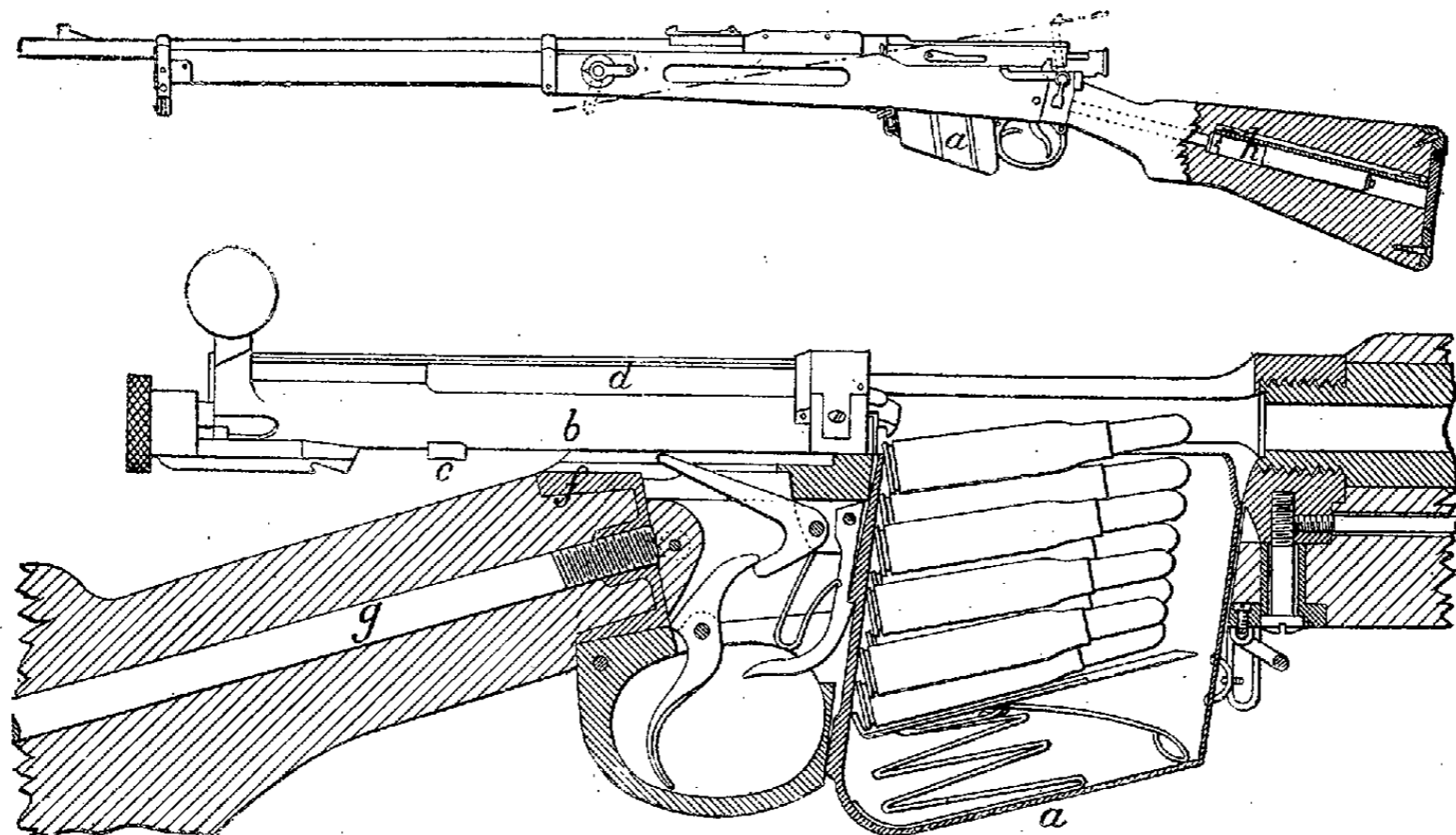
Fig. 14. — Fusil anglais Lee-Metford, modèle 1889.
