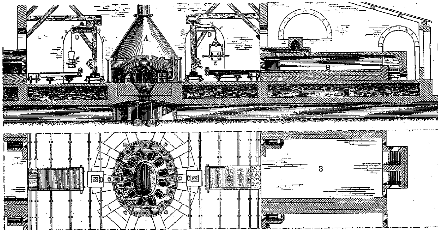
Ensemble de l'installation d'un four de glacerie chauffé à la houille.
