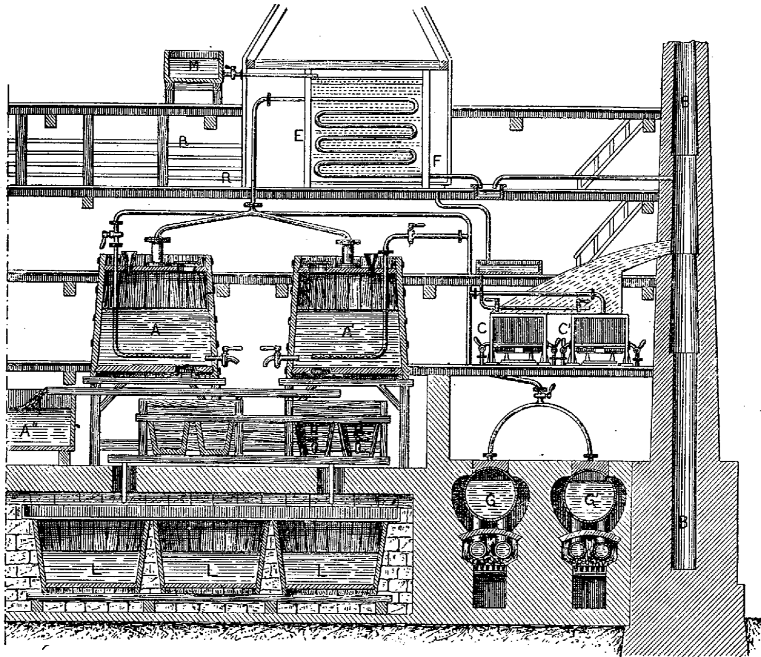
Fig. 1. — AA', cuves d'eau acidulée ; BB, cheminée ; GG', générateurs ; LLL, réservoir recevant la liqueur filtrée ; CC, chaudières de concentration ; HH, filtres ; M, réservoir recevant la liqueur filtrée des réservoirs LLL au moyen d'un monte-jus ; RR, tablettes en plâtre recevant le sucre égoutté ; A'', bassin de dépôt de la liqueur clarifiée ; EF, serpents.
