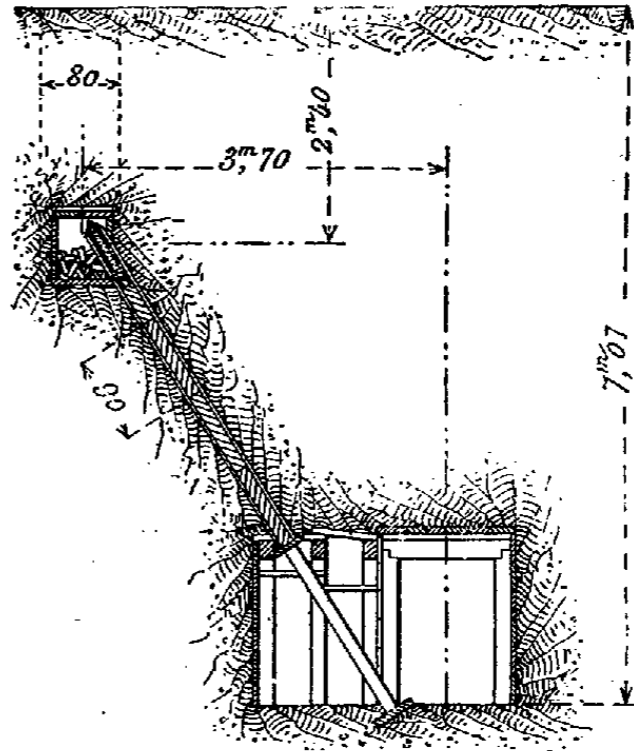
Fig. 3. — Gaine de chargement.
