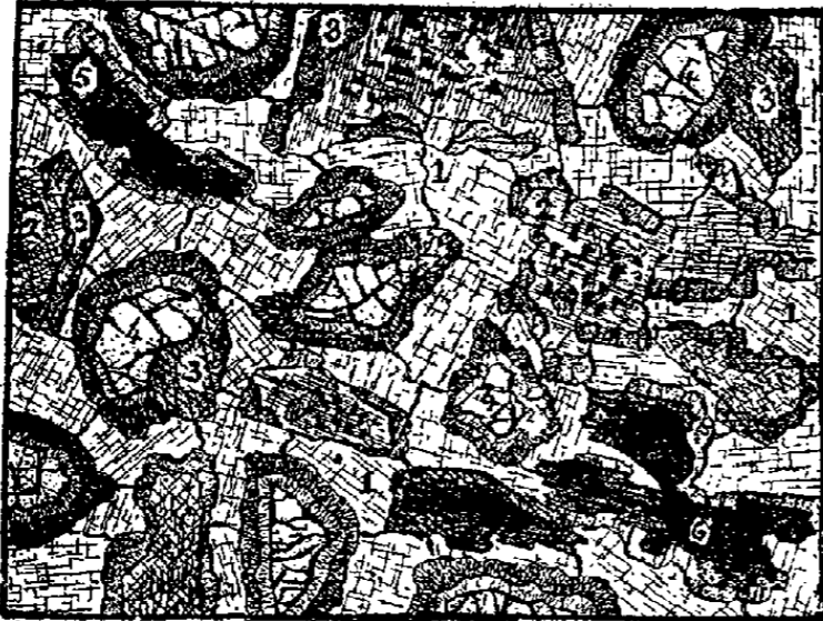
Gabbro à olivine de Pallet (Loire-Inférieure). 1, labrador; 2, diallage entouré d'amphibole brune; 3, 4, olivine entourée d'une double couronne de trémolite et d'amphibole verte; 5, fer titané entouré de biotite; 6, biotite (d'après M. Lacroix).
