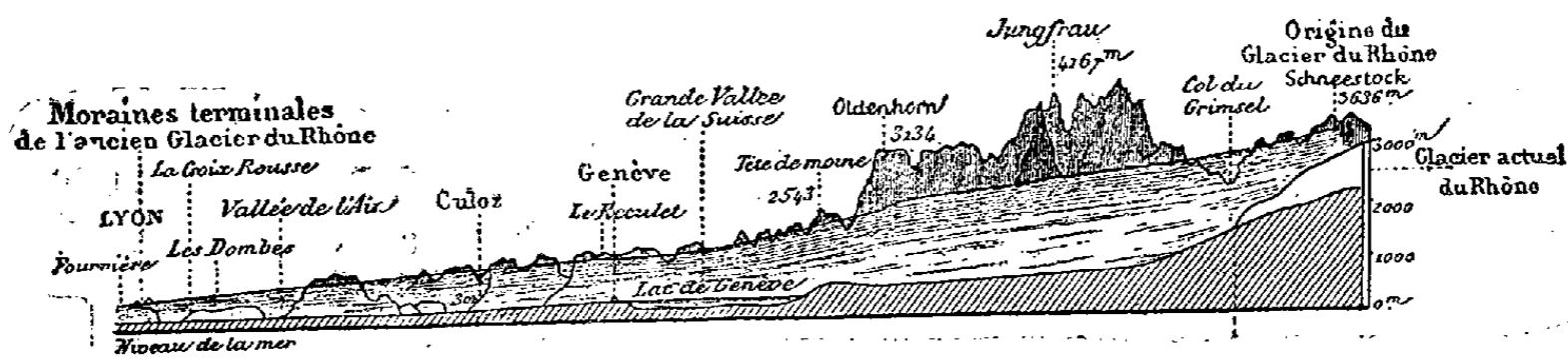
Fig. 17. — Diagramme représentant l'ancienne extension du glacier du Rhône (d'après MM. Chantre et Falsan).
