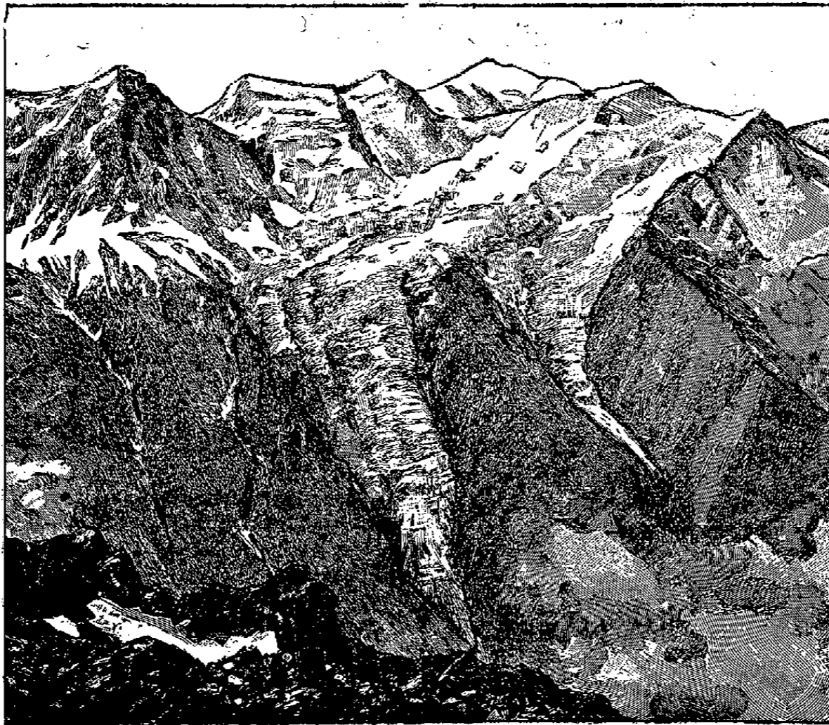
Fig. 4. — Glaciers suspendus du Massif du Mont-Blanc vus du Brevent (d'après nature par M. F. Schrader).
