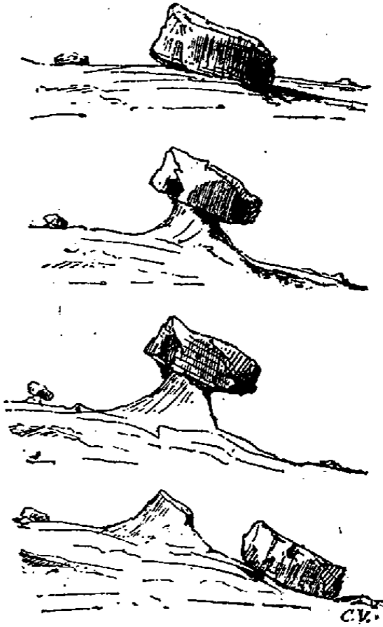
Fig. 9. — Tables de glacier montrant les diverses phases du phénomène qui leur donne naissance, puis motive leur chute.
