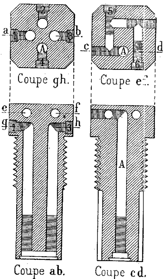
Fig. 3. — Fusée à six durées.
