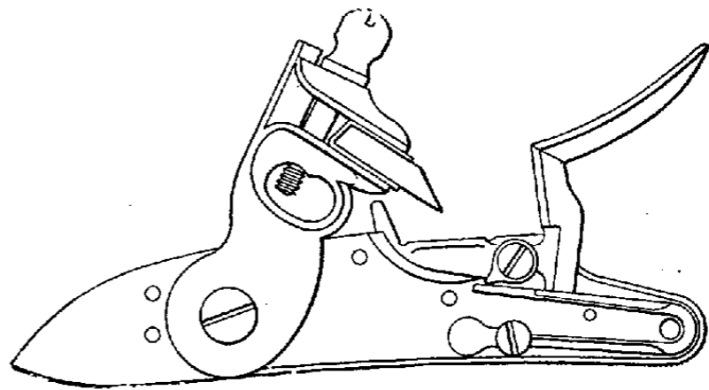
Fig. 7. — Platine à silex (vue extérieure).
