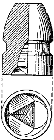
Fig. 9. — Balle modèle 1857.
