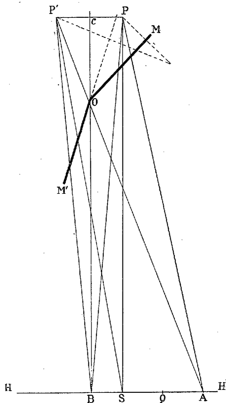
Miroir de Fresnel.
