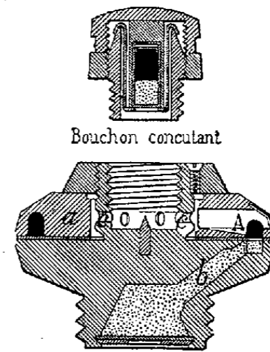
Fig. 6. — Fusée à temps allemande, modèle 1883.
