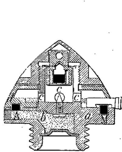
Fig. 5. — Fusée à temps russe, modèle 1888.
