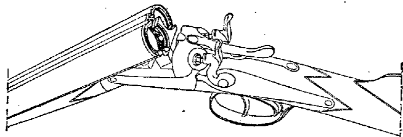
Fig. 20. — Fusil à percussion centrale avec levier top-lever.
