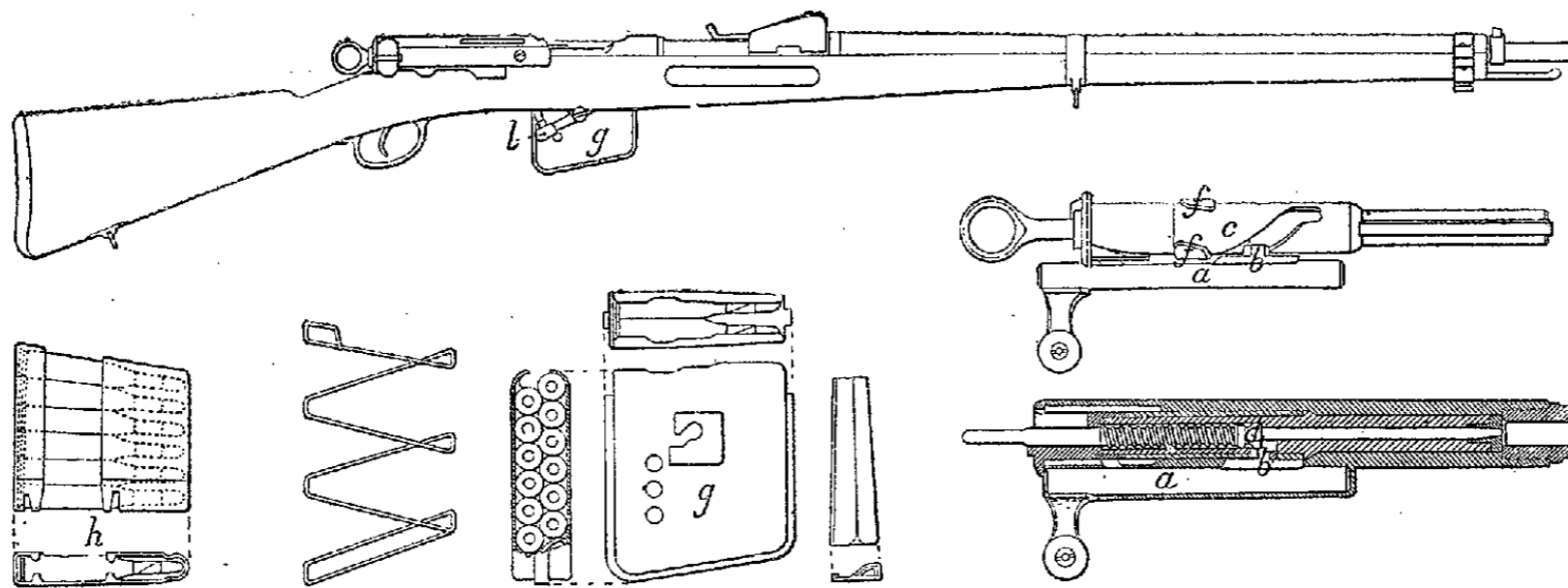
Fig. 18. — Fusil suisse Rubin-Schmidt, modèle 1889.
