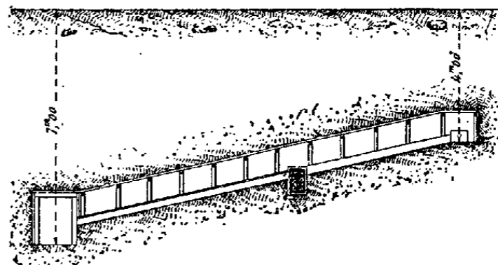
Fig. 4. — Gaine de chargement.
