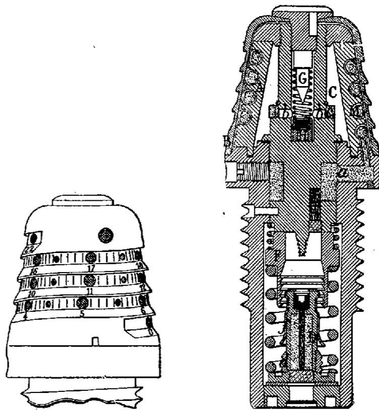
Fig. 7. — Fusée à double effet française, modèle 1884.
