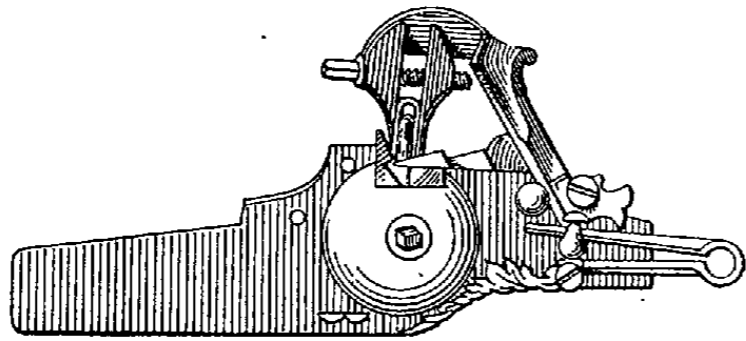
Fig. 6. — Platine à rouet.
