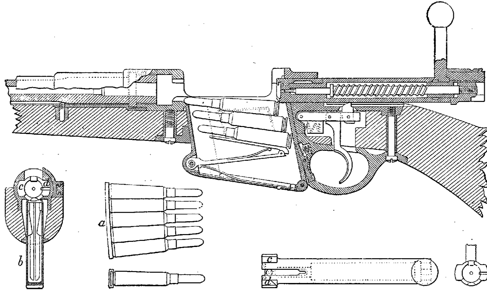
Fig. 16. — Fusil belge Mauser, modèle 1889.
