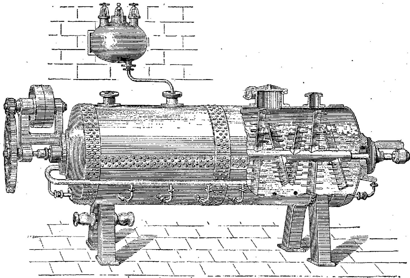
Fig. 2. — Cuiseur-saccharificateur Warein fils et DeFrance.
