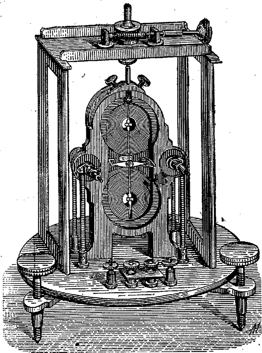
Fig. 2. — Galvanomètre à réflexion de Thomson.
