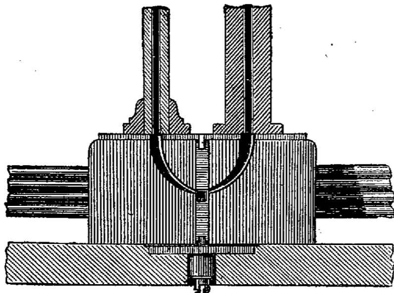
Fig. 4. — Galvanomètre à mercure.
