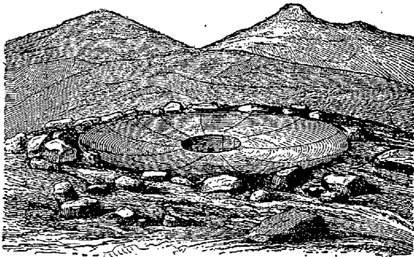
Fig. 3. — Bassin d'un geysir après l'éruption.
