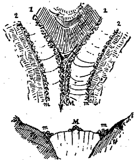
Fig. 10. — Moraine médiane.
